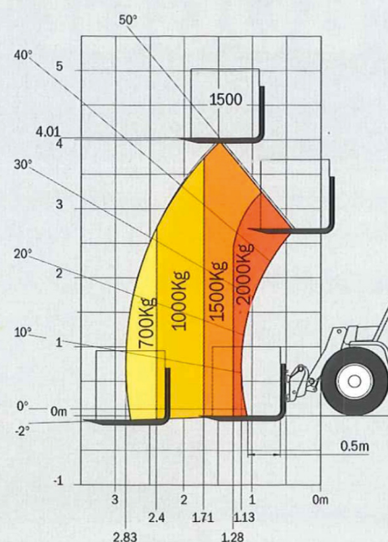
BTI 220 - BT 420 : 2000 kg Tablier à accrochage rapide
